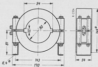
Kabelumbauwandler 7XR9 602
