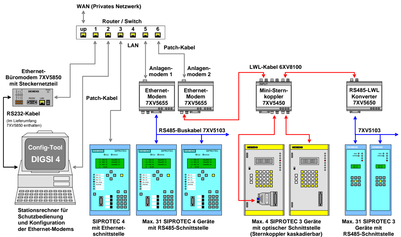
Bild 2 : Anwendungsbereich in Schaltanlagen
