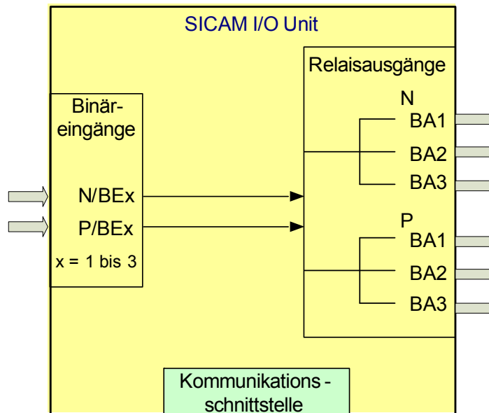
Bild 9-3 Anwendung Kontaktvervielfacher
