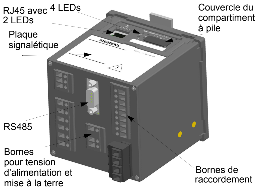
Figure 7-1 Côté bornes, SENTRON T avec RS485
