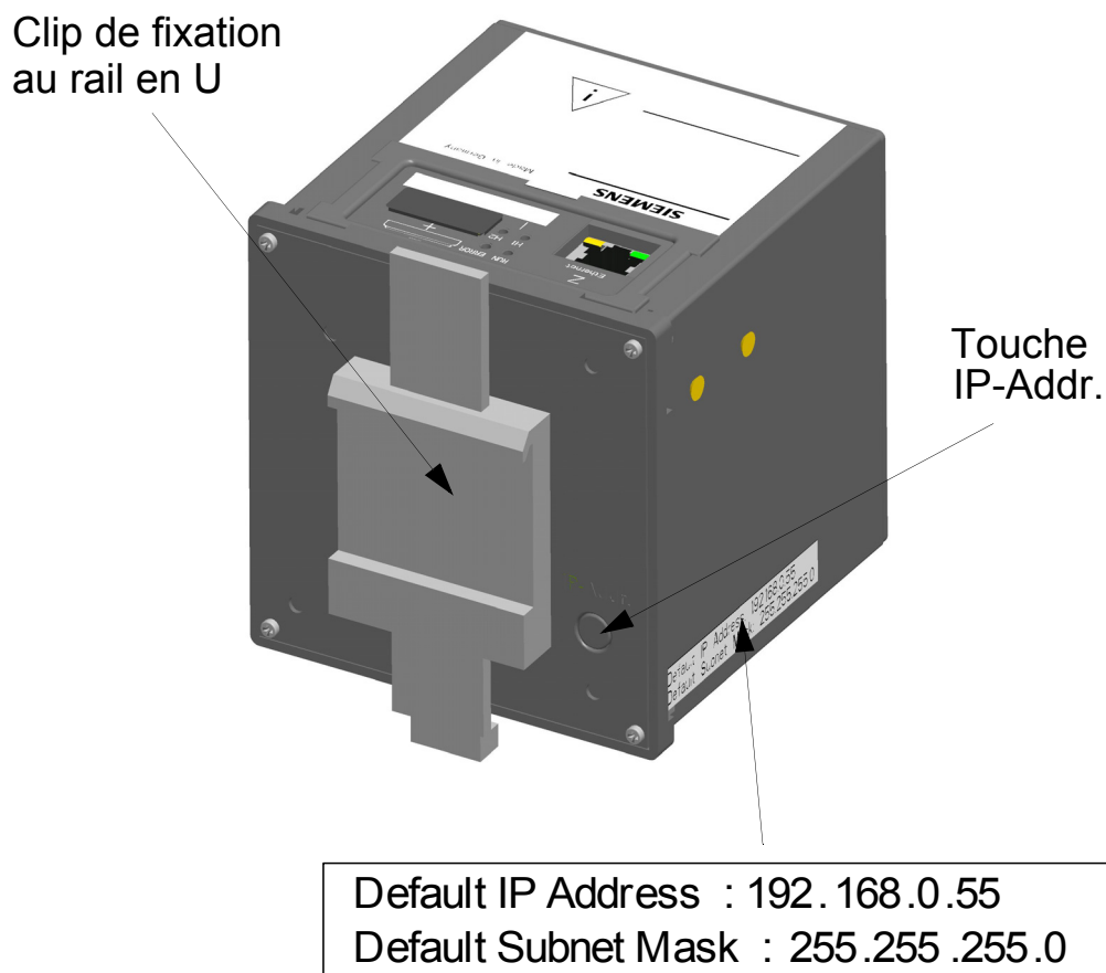
Figure 7-2 Côté rail en U du SENTRON T 7KG966
