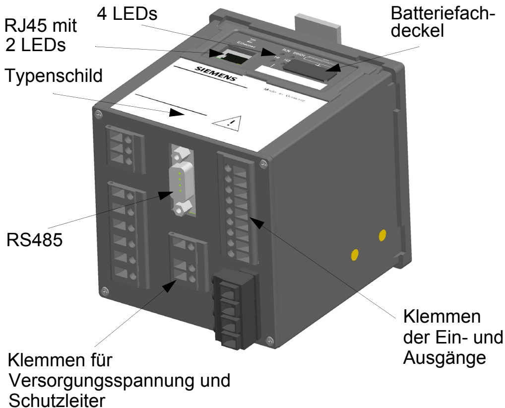
Bild 7-1 Klemmenseite, SENTRON T 7KG966 mit RS485
