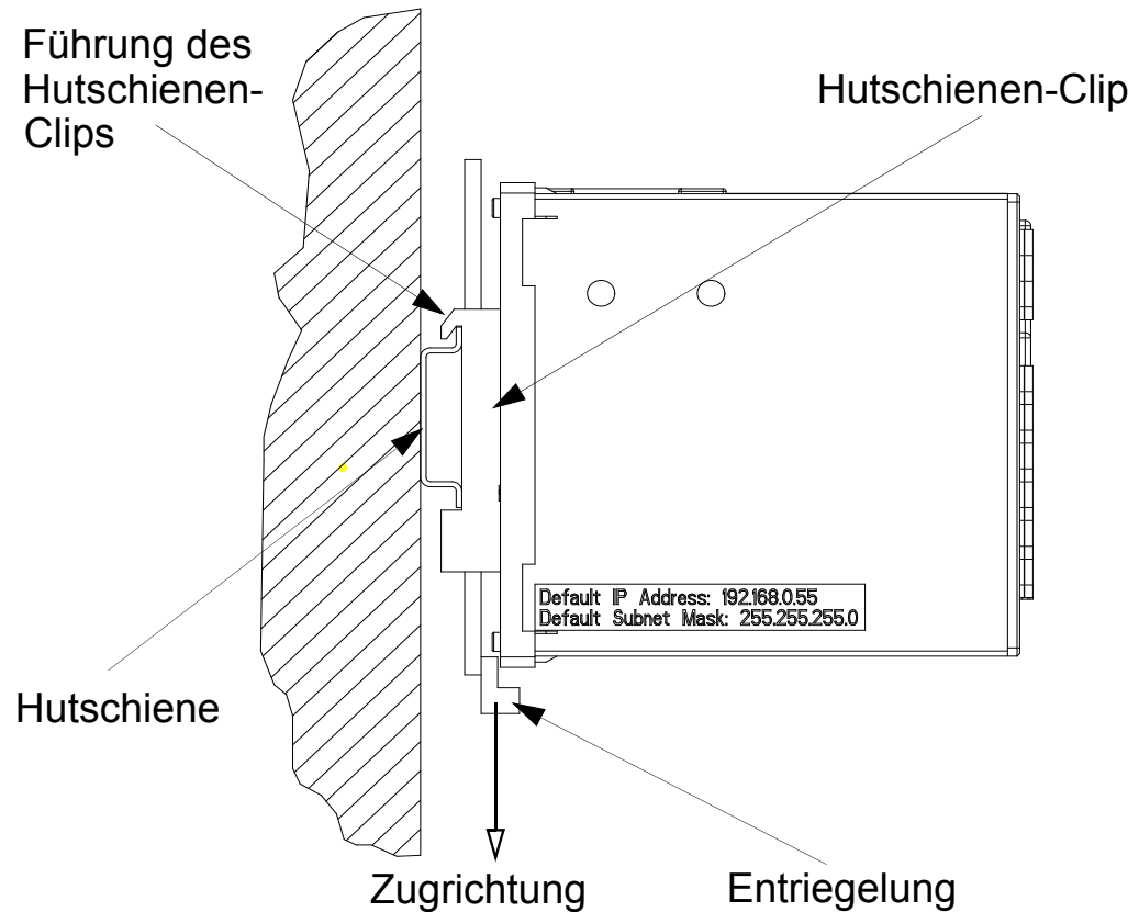
Bild 8-1 Montage auf einer Hutschiene
