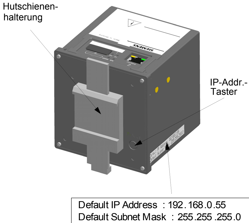
Bild 7-2 Hutschienenseite des SENTRON T 7KG966
