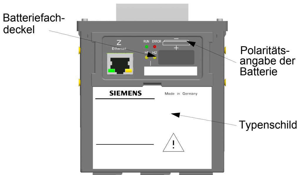
Bild 8-2 Geräteoberseite
