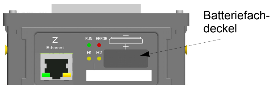
Bild 13-1 Entfernen des Batteriefachdeckels
