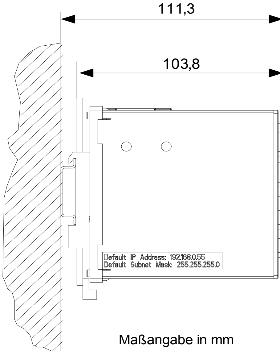
Bild 17-1 Abmessungen
