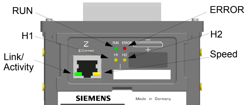
Bild 14-1 Bezeichnung der LEDs
