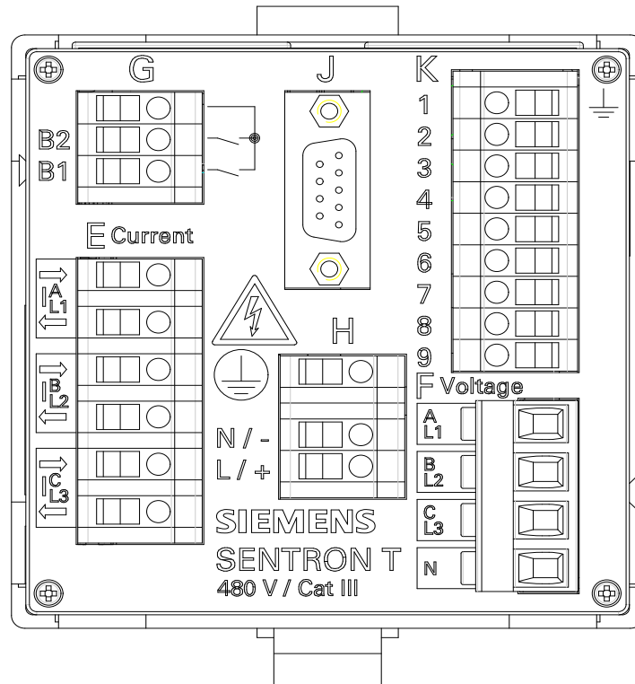
Bild 11-1 Anschlüsse an der Klemmenseite
