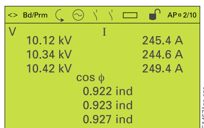
V, I, cos φ (SIMEAS P50)
