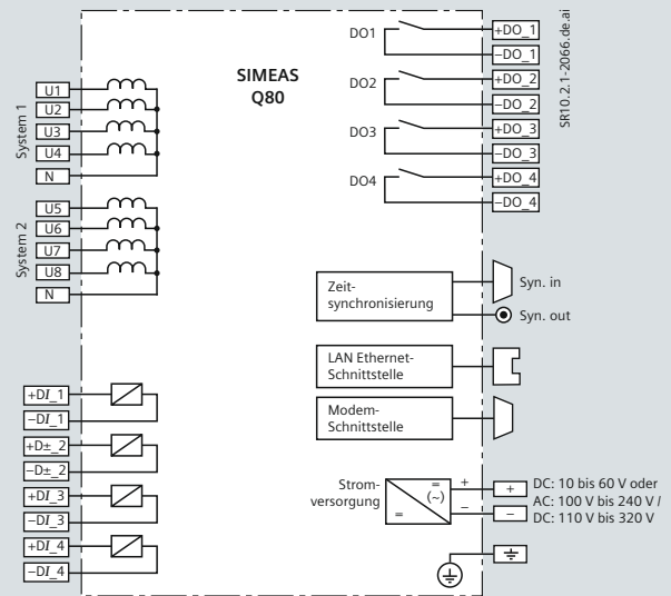
Bild 31 7KG8080 – Acht-Volt-Konfiguration
