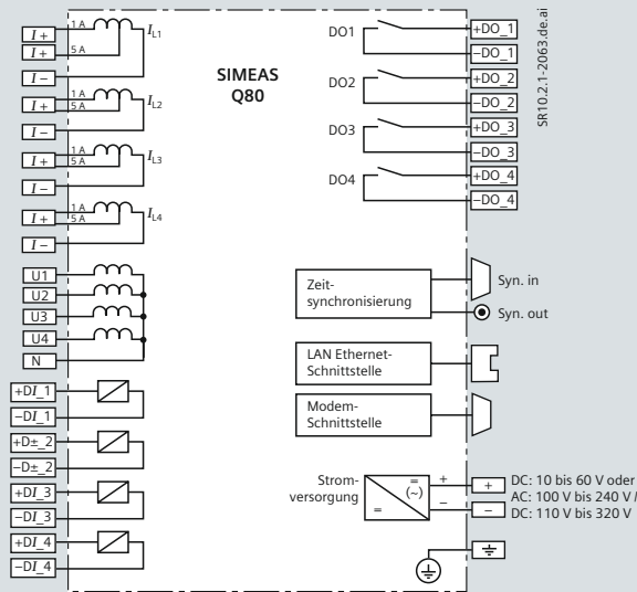
Bild 28 7KG8080 – Vierleiter-Konfiguration
