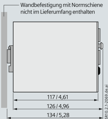
Bild 30 7KG8080: Seitenansicht
