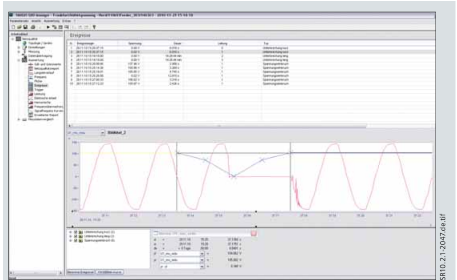
Bild 11 Spannungseinbruch
