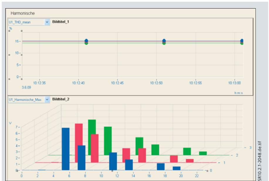
Bild 12 Übersicht Oberschwingungen
