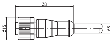
Cavo M12 presa assiale, 3/4/5 poli K-D M12A-...-PVC
