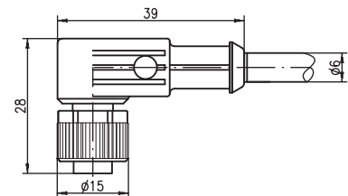
Cavo M12 presa a gomito, 3/4/5 poli K-D M12W-...-PVC
