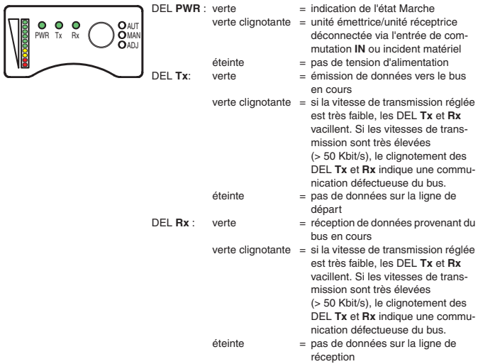
Figure 4.2 : Éléments d'affichage / de commande variante PROFIBUS
