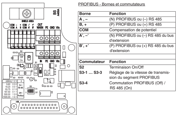
Figure 4.1 : Platine des connexions variante PROFIBUS
