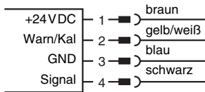
Bild 4.2: Anschlussbelegung M8-Steckverbinder des VARIO B-Lichtvorhangs
