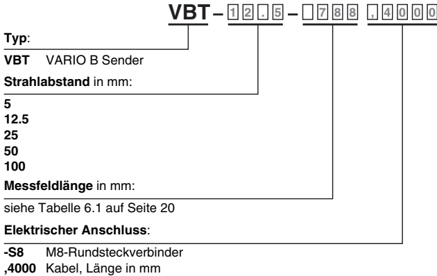
Bild 6.1: Typenschlüssel VARIO B Sender
