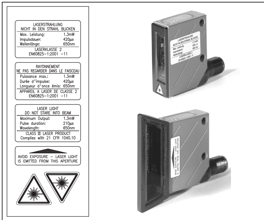
Рис. 2.1: Размещение предупреждающих указателей на корпусе BPS 8
