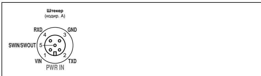
Рис. 3.3: BPS 8 - схема контактов штекерного разъема M12 PWR IN
