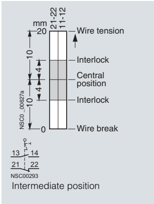
3SE7 140-1BF00
