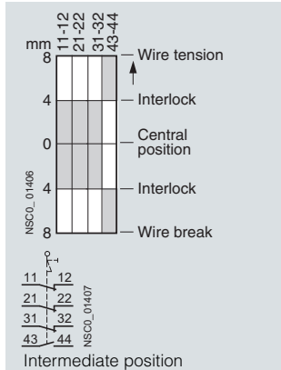
3SE7 141-1EG10
